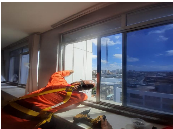
INSTALAÇÃO DE ESTRUTURA EM ACM NOS ACABAMENTO DAS FACHADAS NORTE E SUL
