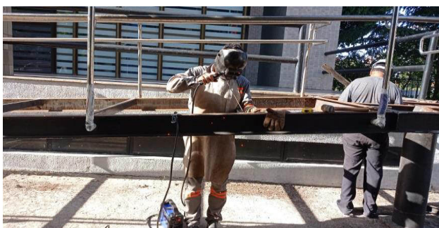
FOTO 11 - Corte e soldagem dos perfis tipo "U" novos.
