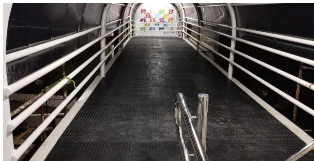
FOTO 15 - Aplicação do piso de borracha da passarela .
