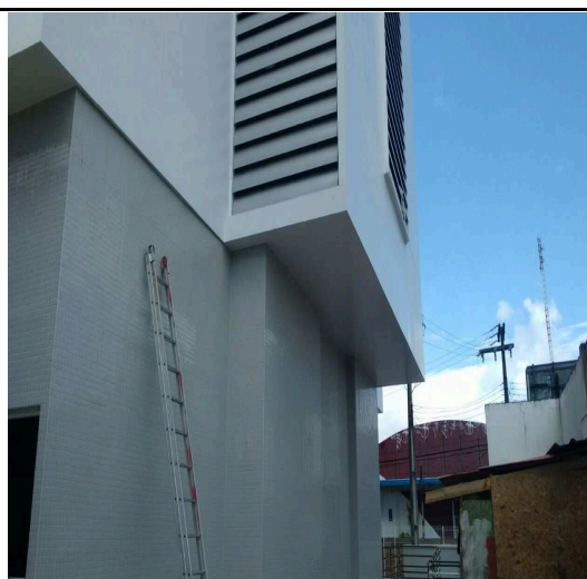
v) DETALHE DE INSTALAÇÃO DOS BRISES DA FACHADA OESTE
