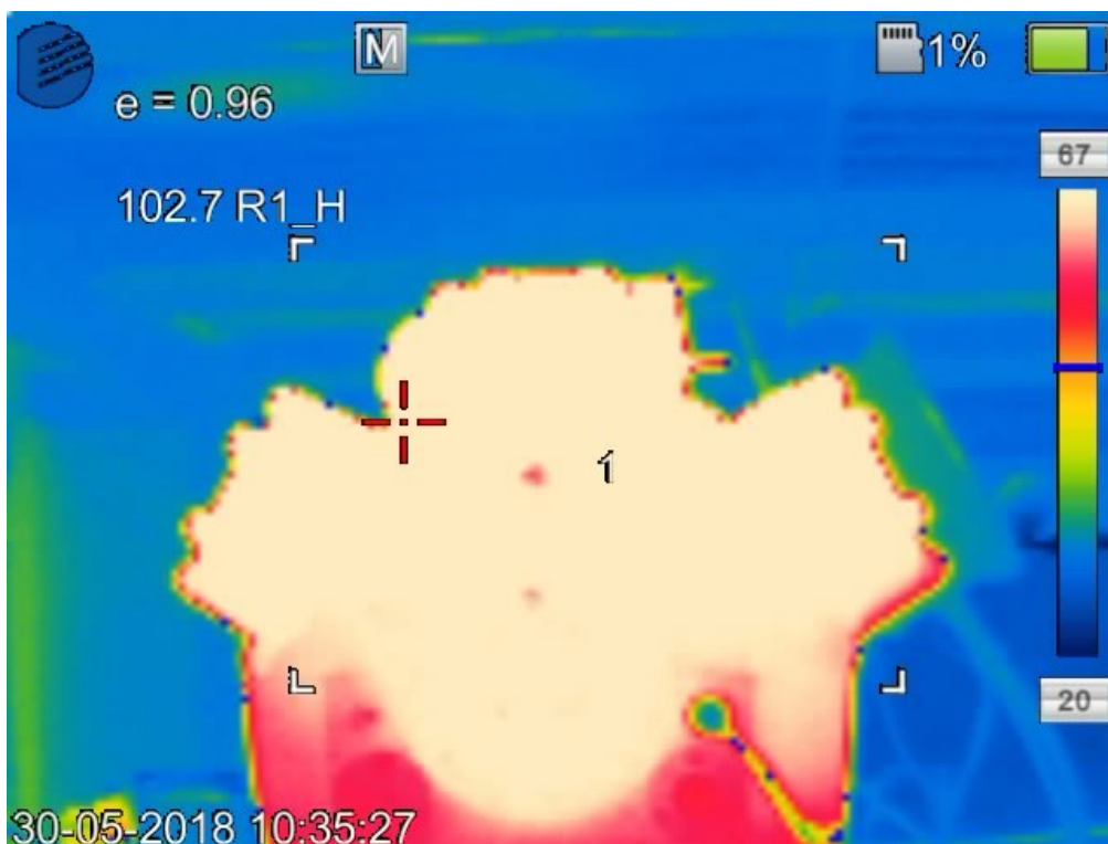
Figura 6 – Termografia evidenciando o sobreaquecimento no compressor COMP6B1.
