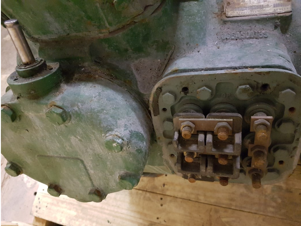
Figura 4 – Caixa de ligação do compressor COMP5A2.
